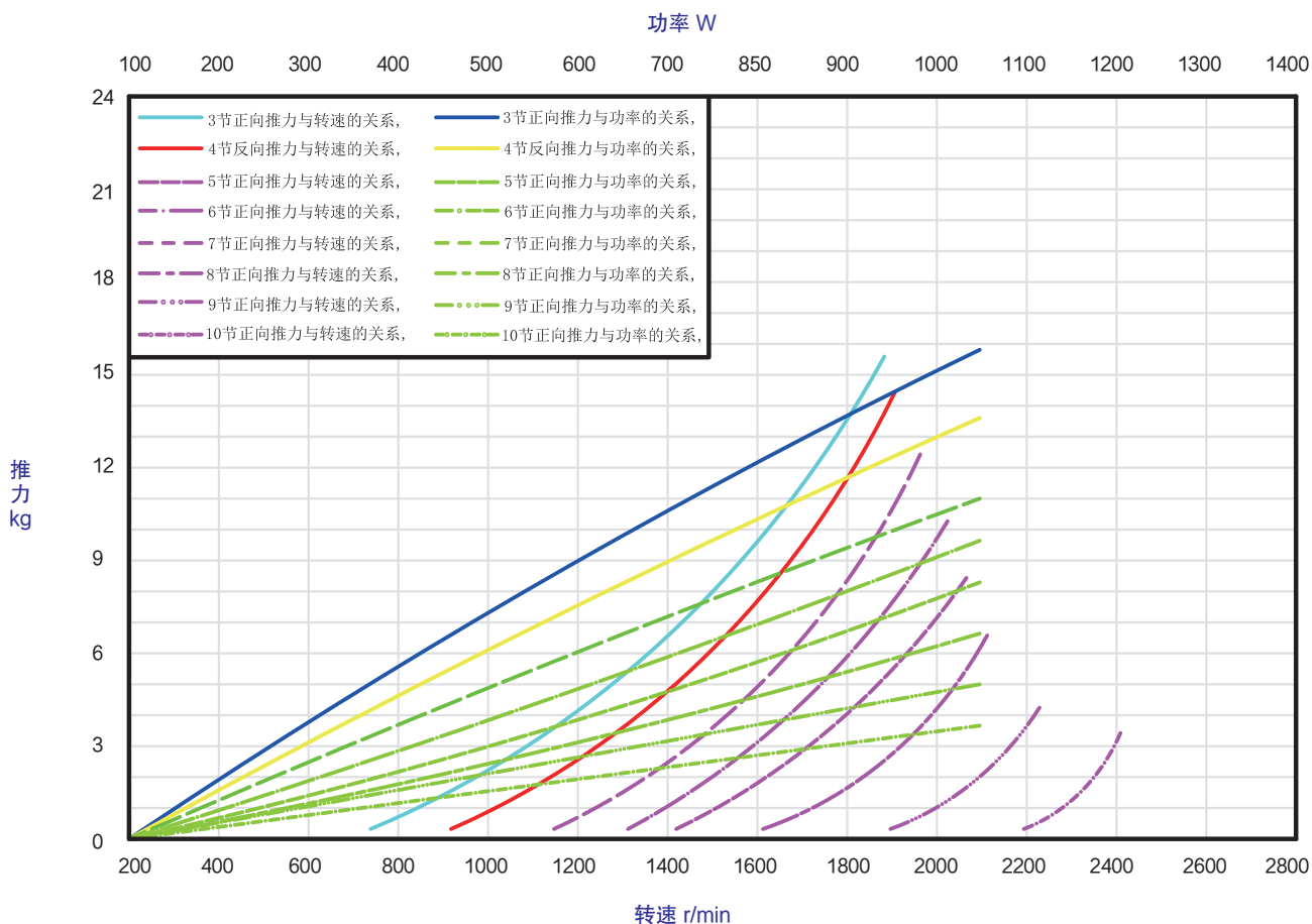
推力与螺旋桨转速关系 &amp; 推力与输入功率关系
