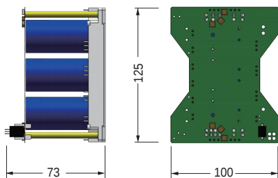
外置驱动版产品外形尺寸
