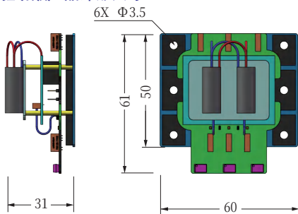
外置驱动版产品外形尺寸
