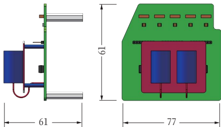
外置驱动版产品外形尺寸
